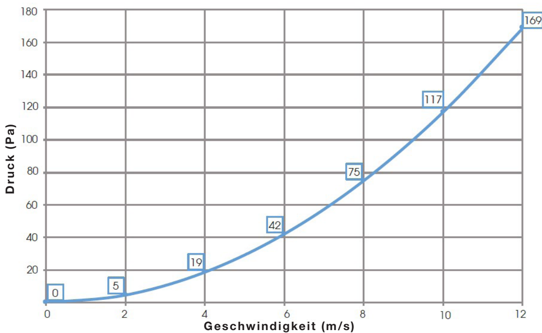
Druckverlustdiagramm
